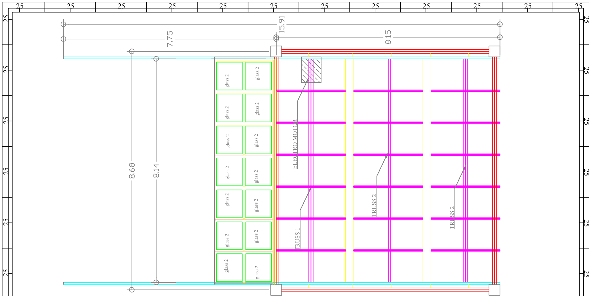
TRUSS PLAN SC : 1/150
